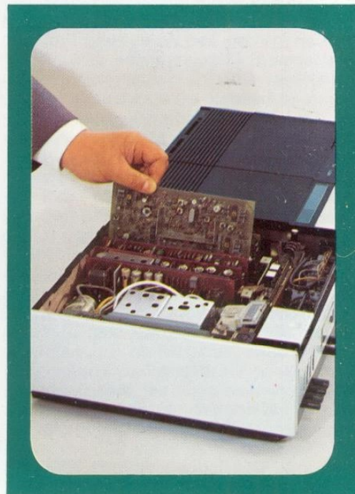
Modultechnik mit sechs steckbaren, schnell austauschbaren Funktionsgruppen.
